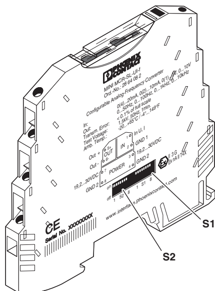
Fig. 7 Position des sélecteurs de codage (DIP)
