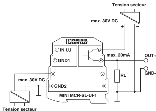
Fig. 1 MINI MCR-SL-UI-F...
