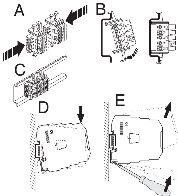
Fig. 4 Montage et démontage
