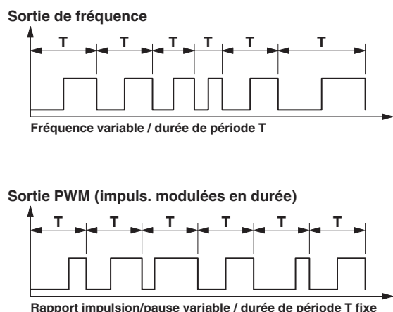
Fig. 8 Signaux de sortie
