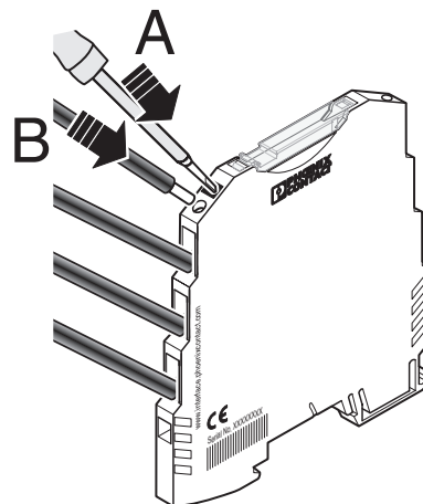
Fig. 6 Raccordement à ressort
