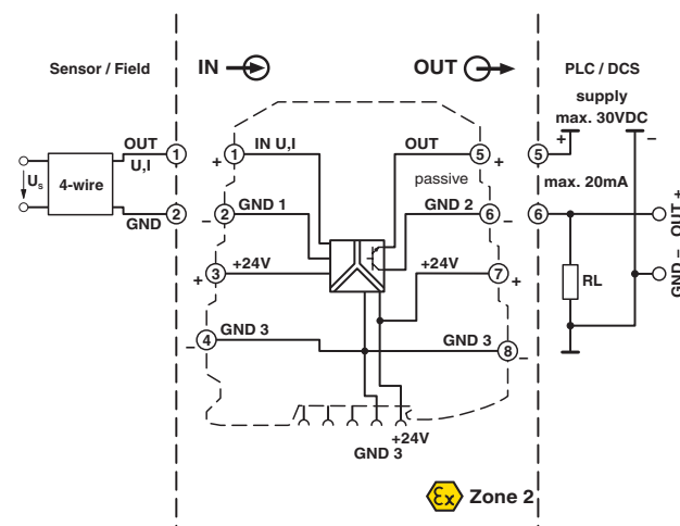
Fig. 3 Diagramme schématique
