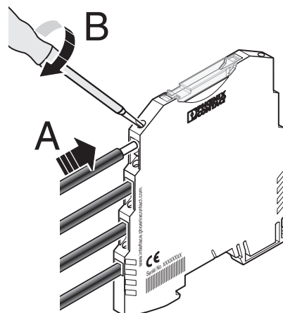
Fig. 5 Raccordement vissé
