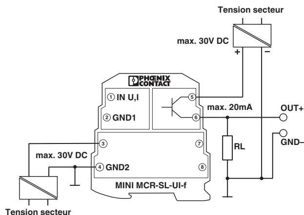
Fig. 9 MINI MCR-SL-UI-F...
