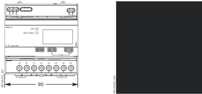
Dimensions de la série iEM3000/iEM3200
