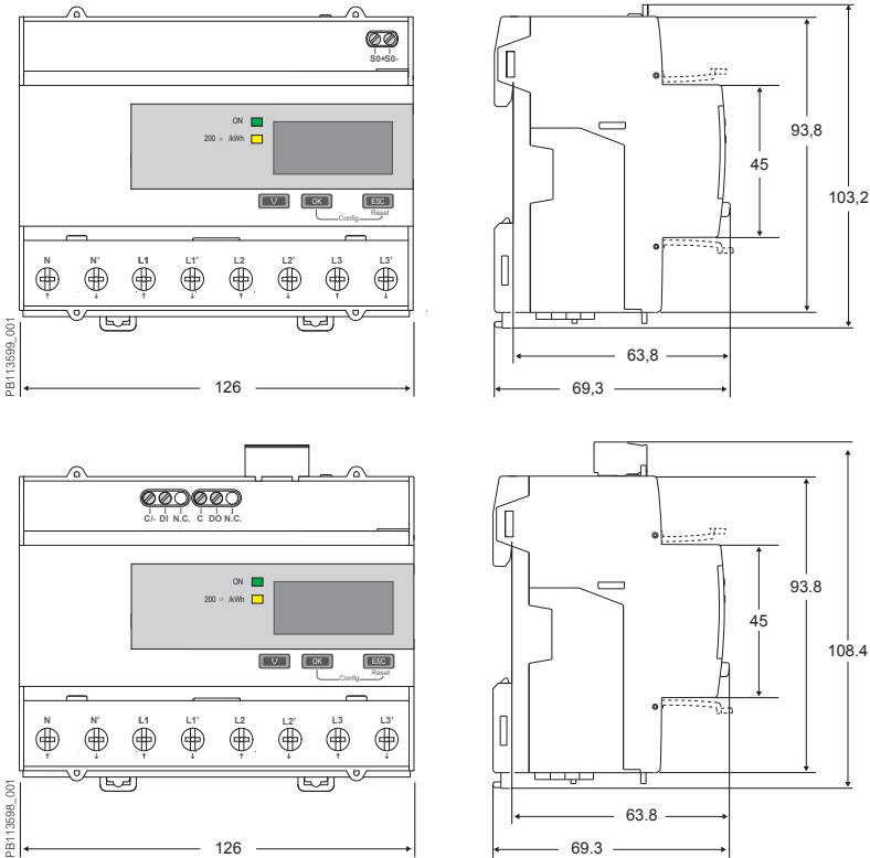
Dimensions de la série iEM3300
