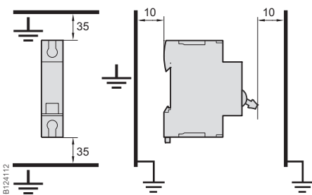
Distances minimales entre le disjoncteur et les parties métalliques reliées à la terre, pour une installation hors enveloppe.
