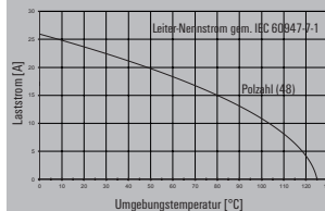
HDC MHE 4X2 FP mit HDC MHE 4MP / H07V-K2,5
