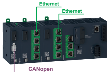
Contrôleur logique Modicon M262 avec 3 modules de communication intelligents TMSES4 et TMSCO1 (TMSCO1 : toujours le module le plus à gauche) : configuration maximale avec CANopen
