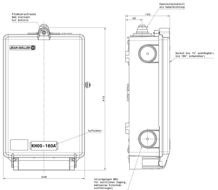
Ansicht ohne Deckel und Abdeckungen
