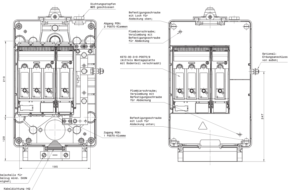
Ansicht ohne Deckel und Abdeckungen
