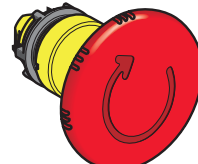
Tourner pour déverrouiller (EN/ISO 13850) ZB5AS8/4 voir page 41
