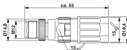
Dessin coté
