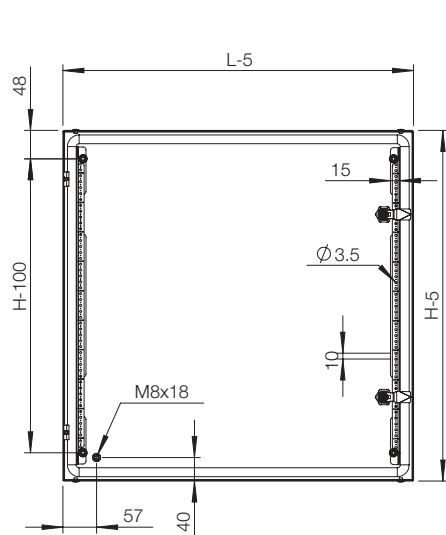
Vue de la porte intérieure
