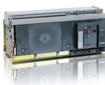
Masterpact NW 4000... 6300 A Courants de court-circuit: 100 / 150 kA
