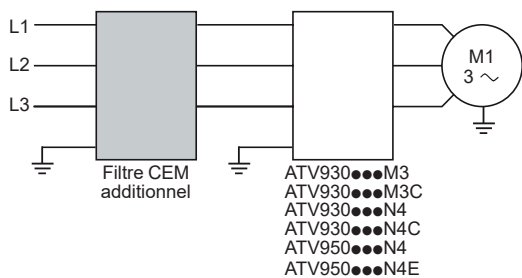
Variateur Altivar Process avec filtre CEM additionnel
