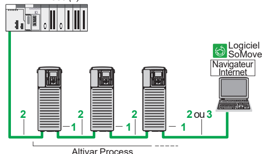
Exemple de raccordement sur réseau Ethernet/IP
