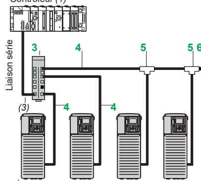
Altivar Process Exemple d'architecture liaison série
