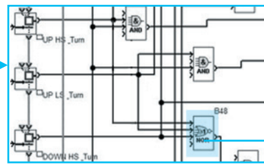
3 Suppression du bloc "OR" et positionnement du bloc "NOR" en lieu et place
