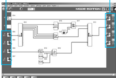
Fenêtre d'Édition de programme FBD
