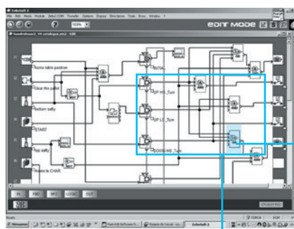
1 Bloc "OR" à remplacer
