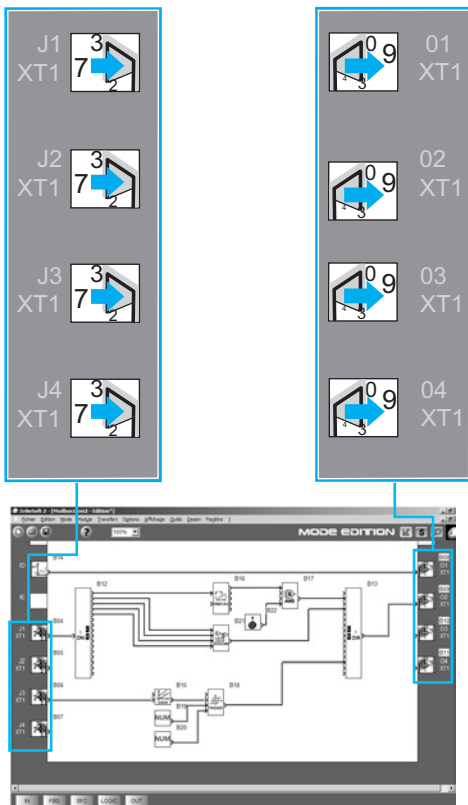
Fenêtre d'Édition de programme FBD
