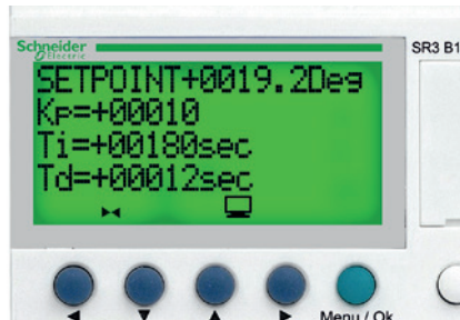
Modification des paramètres (Kp, Ti, Td) avec les touches de programmation et paramétrage
