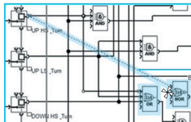
2 Déplacement des liens sur le nouveau bloc "NOR"
