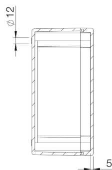
SECTION A-A
