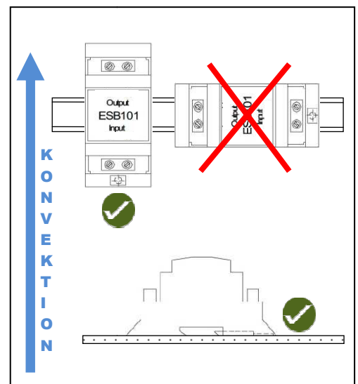
(Abb.10 Montagerichtung)
