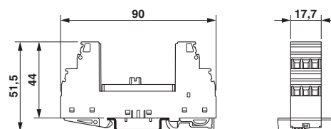
Maßzeichnung
